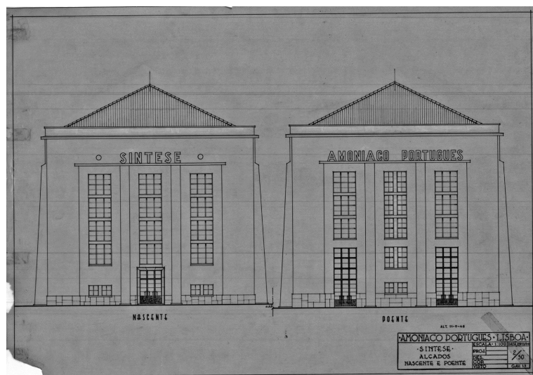
Fig. 6 – Edifício da Síntese I, Alçado Nascente e Poente. Outubro de 1946 Arquivo Quimiparque, Estarreja
