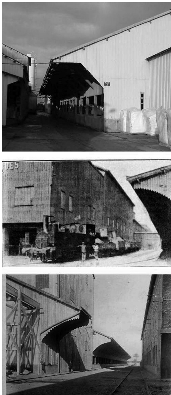
Fig. 3 – A «assinatura» Stinville no pormenor construtivo das abas em Honfleur (estado actual) , La Rochelle (demolida) e Barreiro (demolida), de cima para baixo
