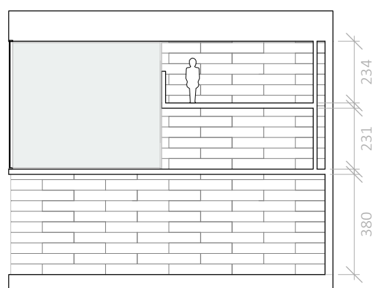
Módulo 2 | Corte
