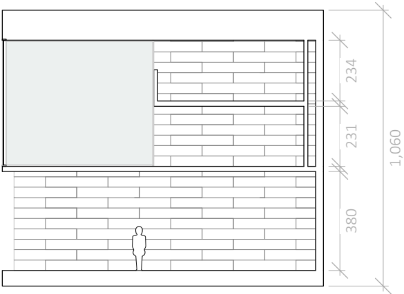
Módulo 1 | Corte
