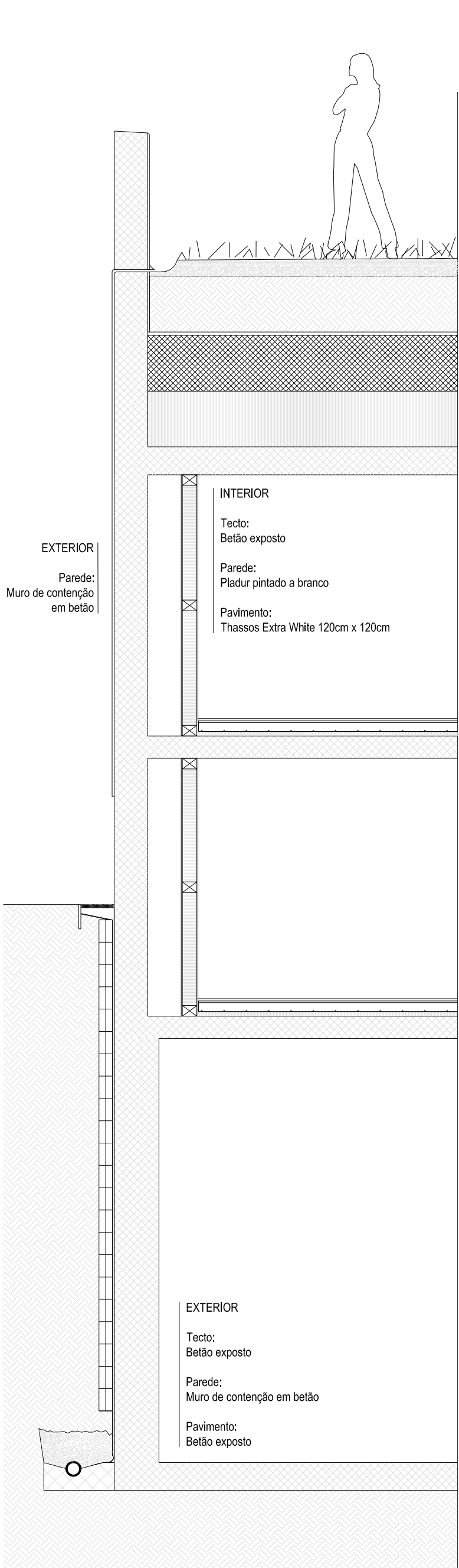
Figura 92 - Corte de materialidade (Escala: 1:40)
