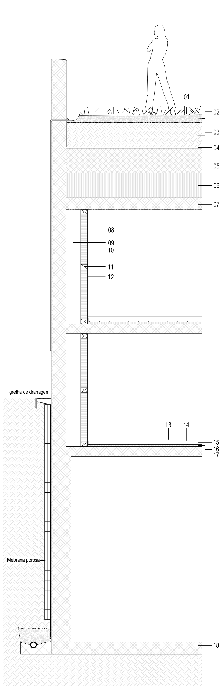
Figura 90 - Corte construtivo (Escala: 1:40)
