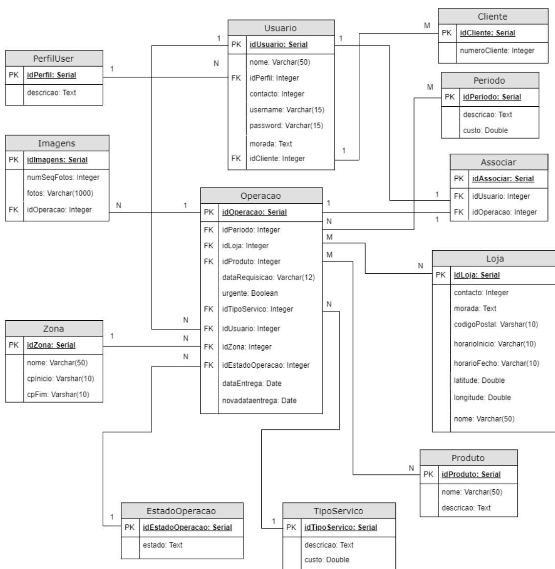
Figura 1 - DER do projeto
